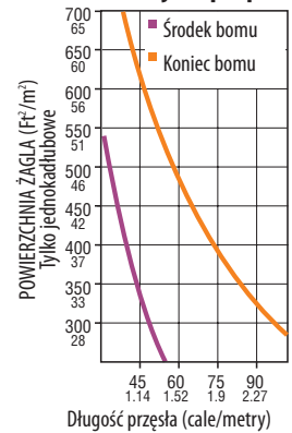
Maks. dł. szyny wyskiej 32 mm mocowanej bez podparcia
