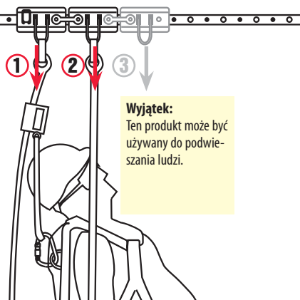
Wózek zaopatrzony w bolce blokujący umożliwia ruch lub zablokowanie na pozycji.
